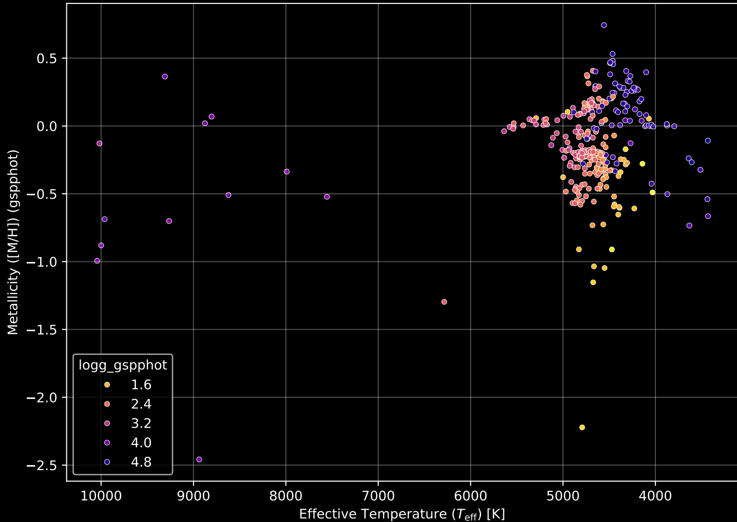
APOGEE DR17 Field: [214+18_btx] Stellar Population Parameters (n= 319)
